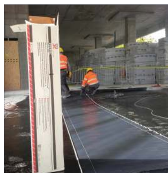
2. Instalacja hydroizolacji Proofex 3000 na patio.
